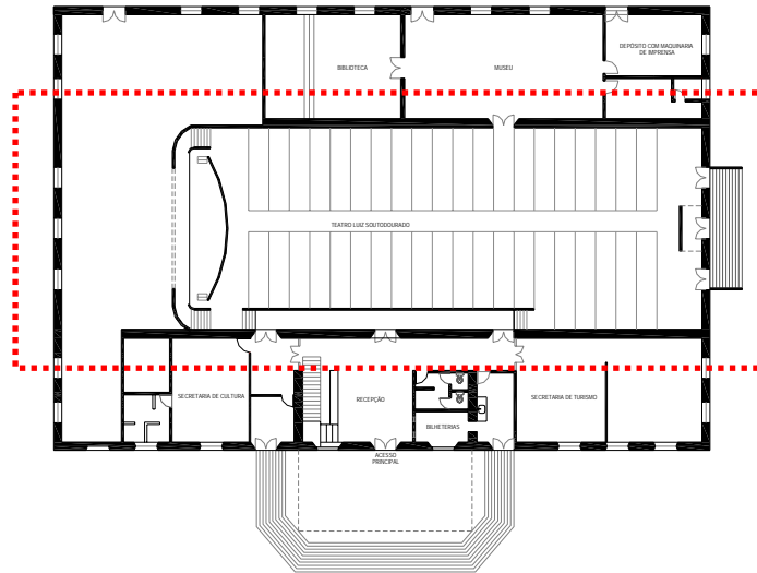
Figura 14: Planta atual da antiga estação. Retirada dos trilhos e inserção do teatro, no módulo central da edificação; sem escala; Fonte: Secretaria de Planejamento de Garanhuns; escadas esquemáticas; elaborado por Daniella Esposito, abril 2009.
